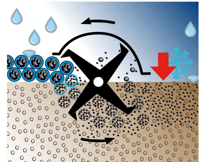
Der hydrophobierte Holcim Hydroport wird erst durch das Einfräsen aktiviert und führt zur gewünschten Bodenverfestigung.
