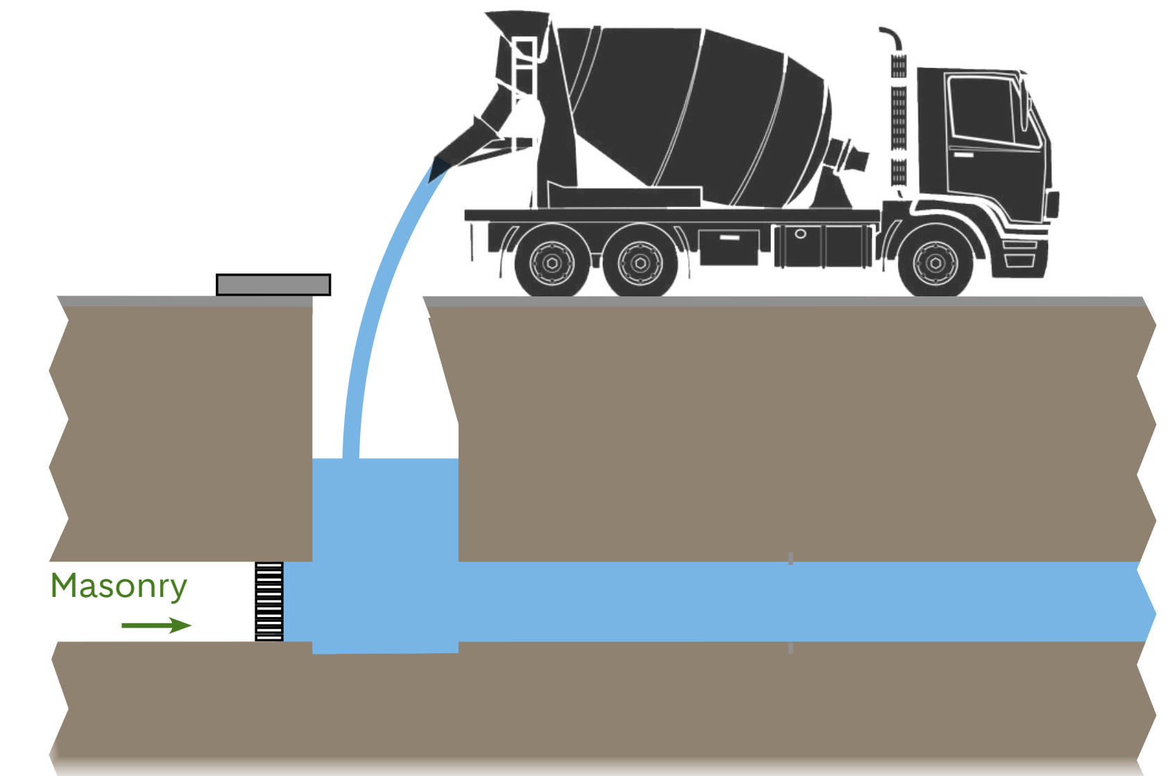
Verfüllung stillgelegter Kanal über Schacht
